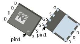
DFN5 x 6
